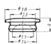
Stopfen
